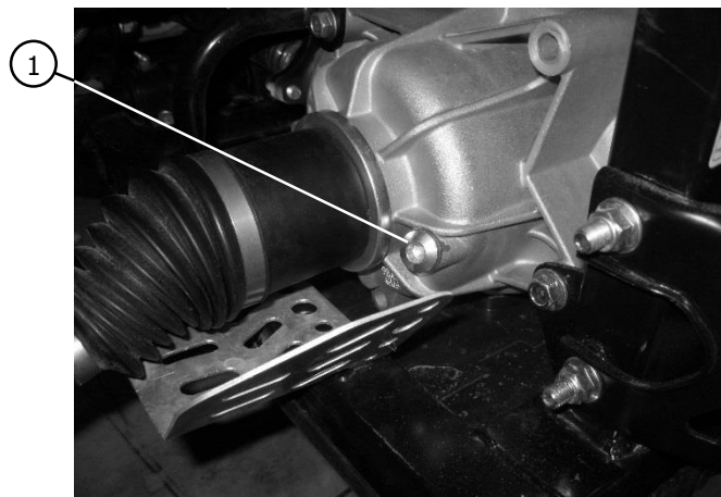
1) Болт заливного отверстия заднего редуктора
